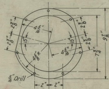
2394 SPECTACLE RING
