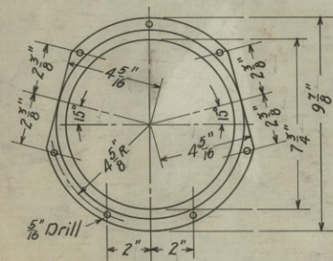
2393 SPECTACLE RING
