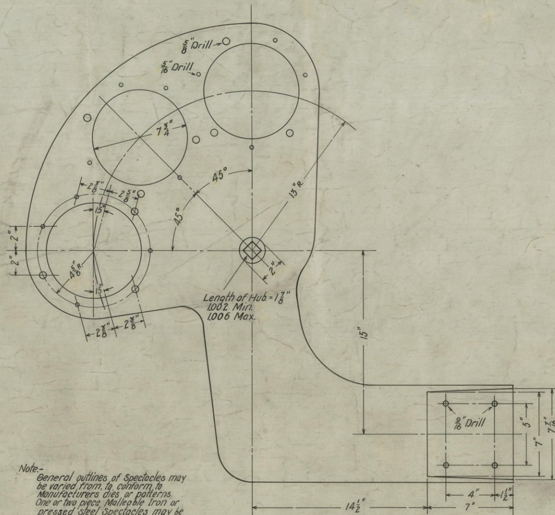
2392 SEMAPHORE SPECTACLE
